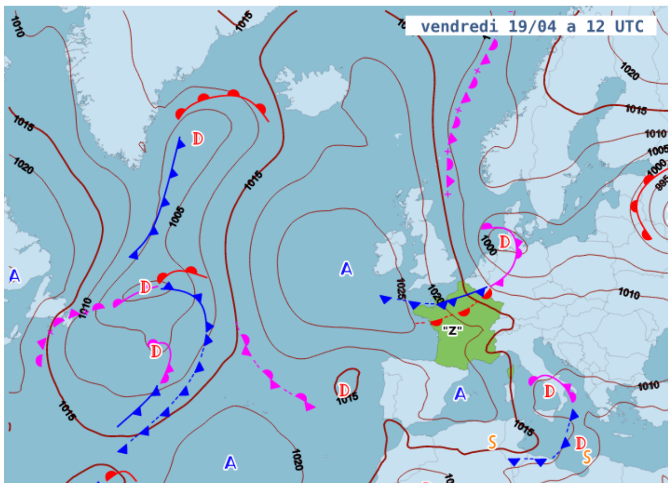
Carte des fronts prévue pour vendredi 19/04 à 14h locales
