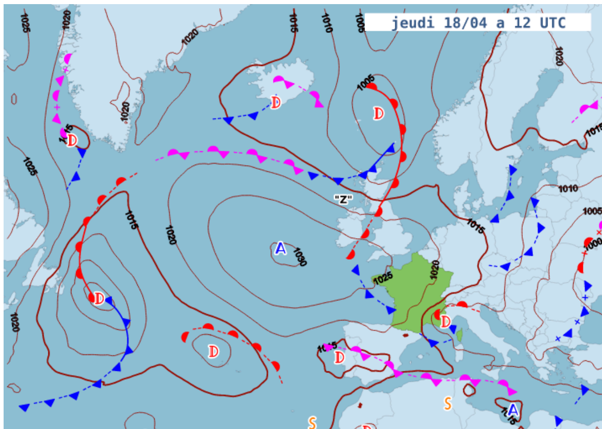
Carte des fronts prévue pour jeudi à 18/04 à 14h locale
