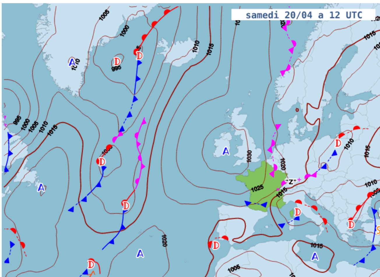
Carte des fronts prévue pour samedi 20/04 à 14h locales
