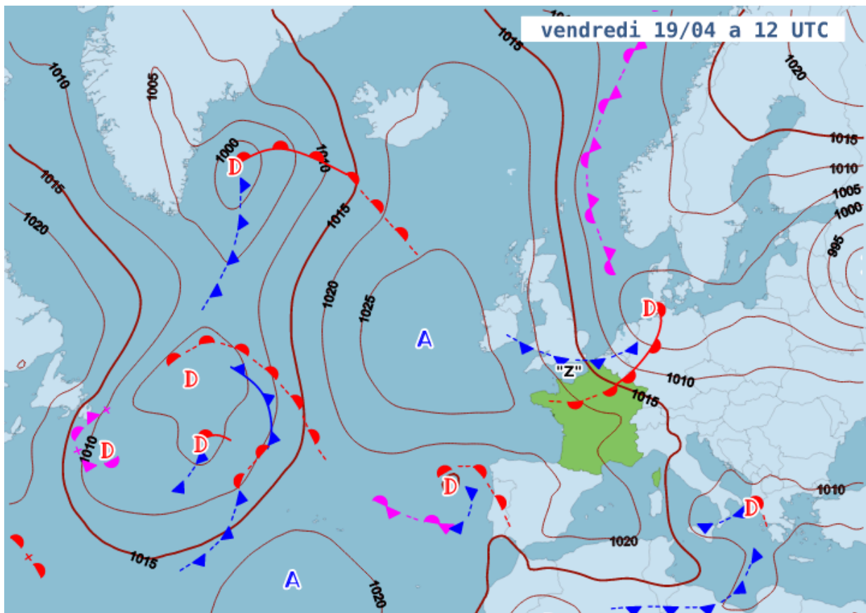
Carte des fronts prévue pour vendredi 19/04 à 14h locales
